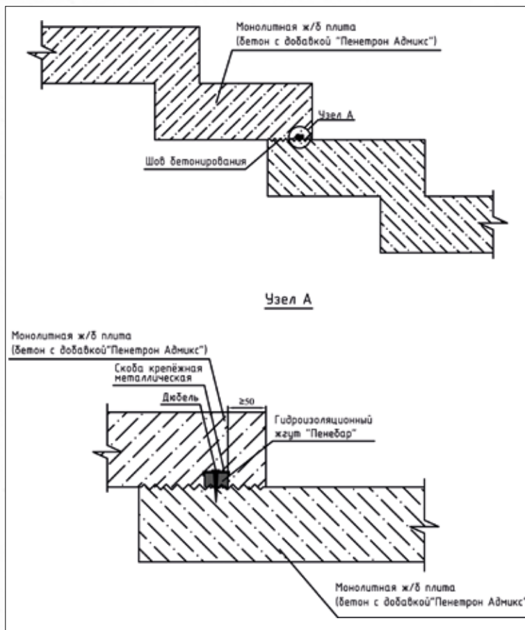
Рисунок 8 – Схема устройства гидроизоляции ограждающих элементов конструкции и швов бетонирования в трибунных перекрытиях при их возведении
