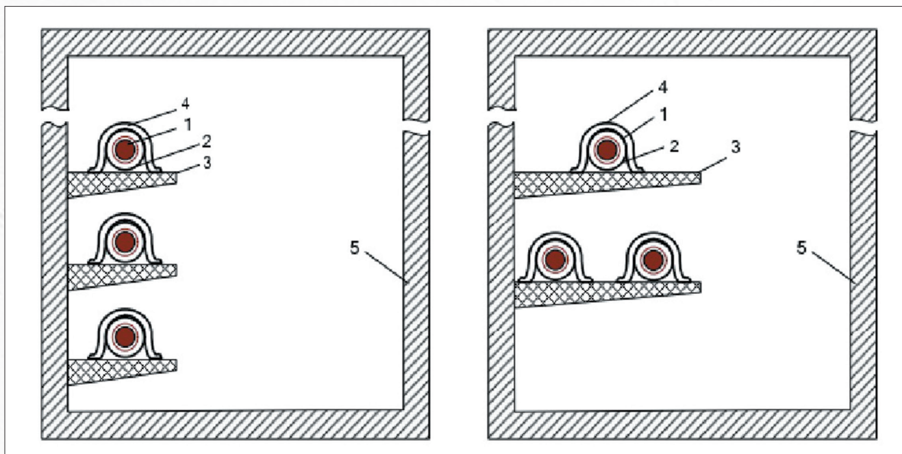
Рис. 1. Различные типы прокладки кабелей в кабельном тоннеле
