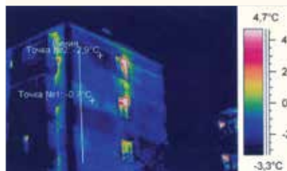
Инфракрасный снимок поверхности стен жилого дома после нанесения Изоллата
